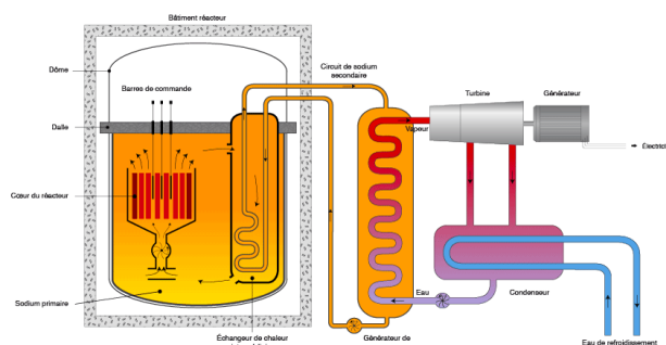
Figure 31 : schéma de fonctionnement d'un réacteur RNR
