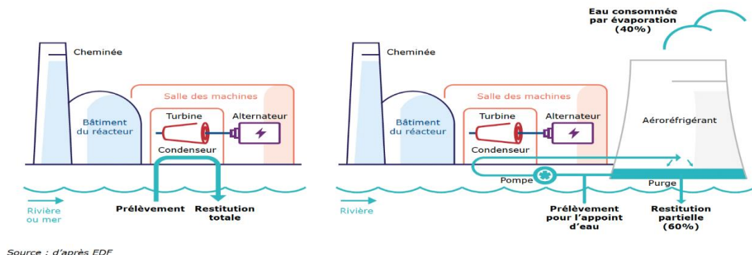
Figure 8.13 Fonctionnement d'une centrale en cycle ouvert (à gauche) et en cycle fermé avec aéroréfrigérant (à droite).
