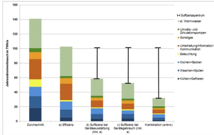
Quantification des effets d'économie d'électricité dans le secteur résidentiel allemand en cas d'exploitation complète des potentiels d'efficacité et de sobriété énergétique. Source et mise en page : Wuppertal Institut .
