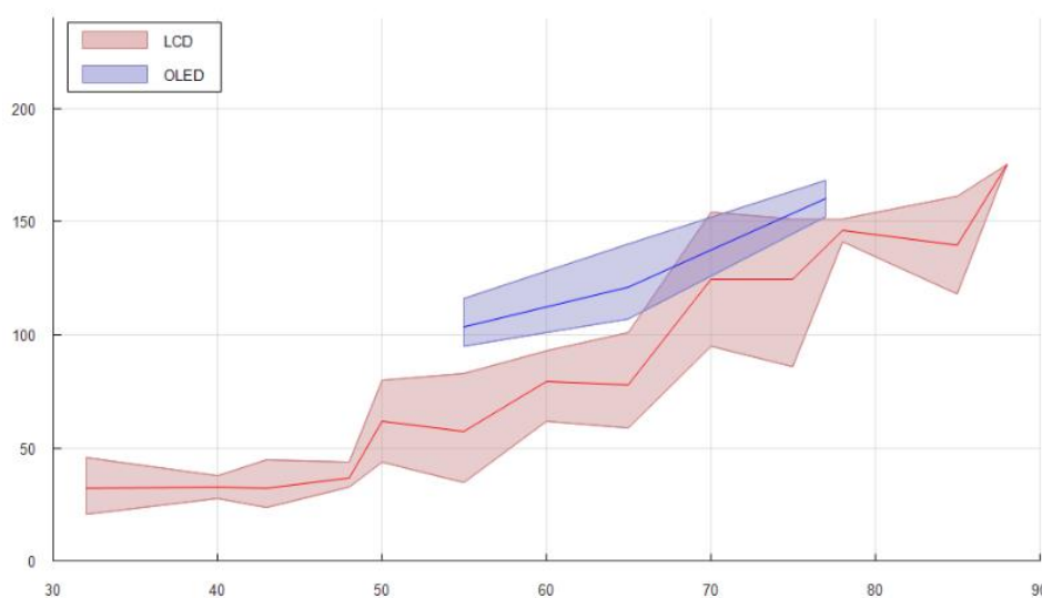
Consommation en watts d'un téléviseur de technologie LCD ou OLED en fonction de sa taille (source : rtngs.com)
