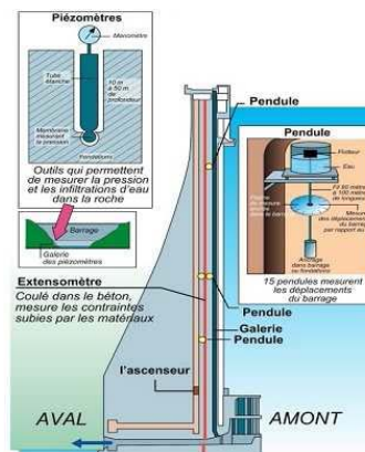
Les outils de l'auscultation - Source : EDF
